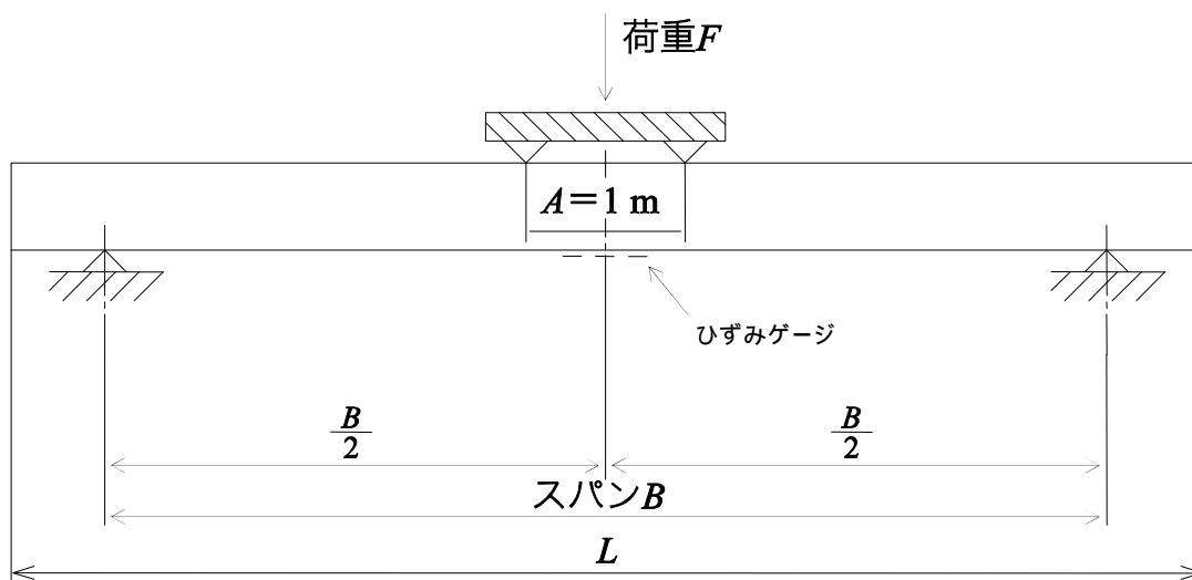
参考図 5 曲げ強度試験の載荷方法
