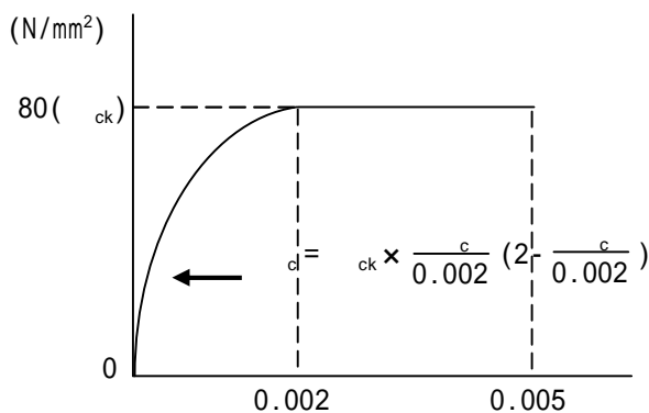
参考図 3 コンクリートの応力度～ひずみ曲線 (土木の場合)
