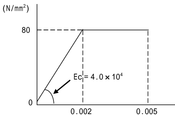
参考図 1 コンクリートの応力度～ひずみ曲線 (建築の場合)
