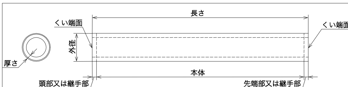
図 1 - SC くいの形状
