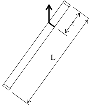
参考図 6 建て込みにおける SC くい の吊り点位置
