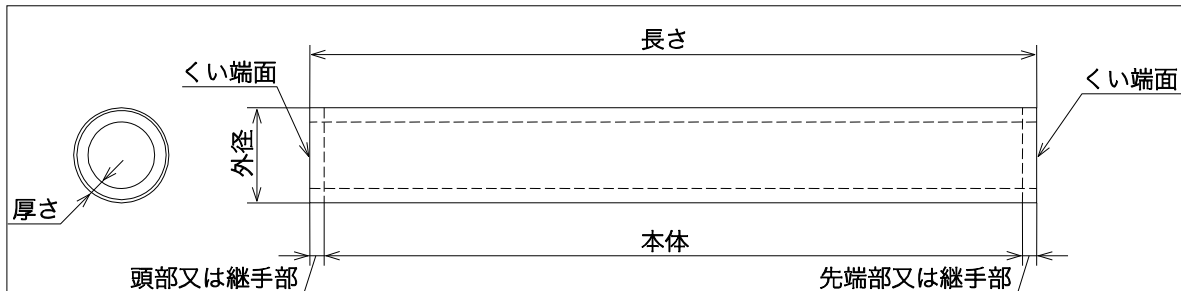
図 1-SC くいの形状
